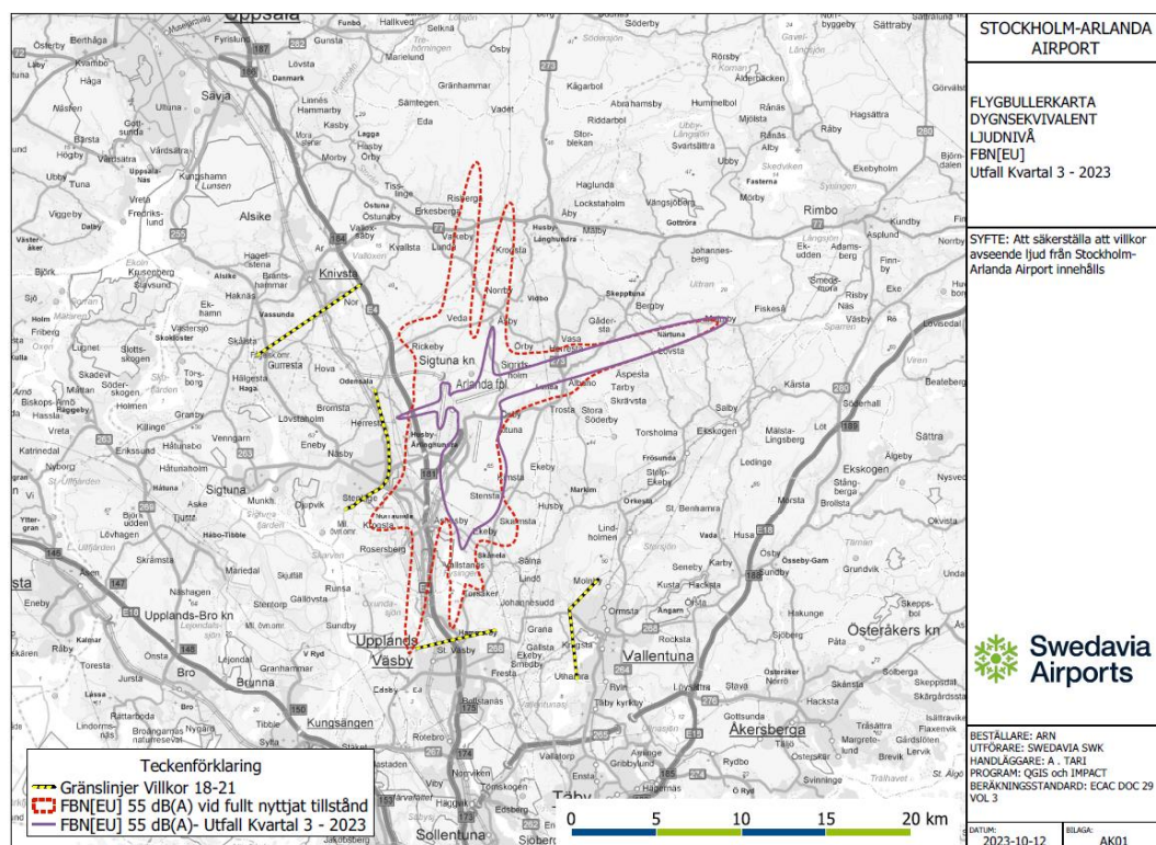
Figur 8. Utfall dygnsvägd ekvivalentnivå 55 dB(A), jämfört med motsvarande gränslinjer streckade i gult. I Figuren visas även FBN 55 för tillståndsgiven trafik i röstreckad kontur.
