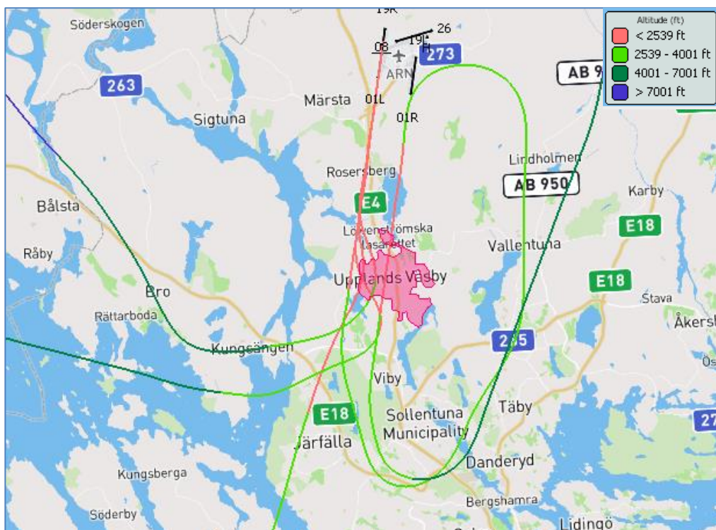
Figur 6. Rörelser som har fastnat i kontrollen för villkor 11 under perioden. Röd del av spåret är under 750 m (MSL).
